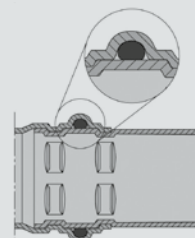
De dubbele persing zorgt voor extra zekerheid.
