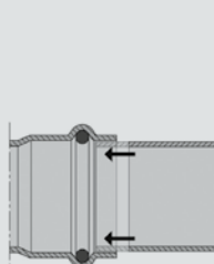
De cilindrische buisvoering beschermt het hoogwaardige dichtelement.
