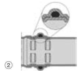
Doorsnede van een geperste fitting.
